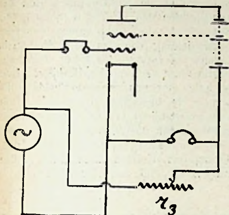
Figuur 8. — Methode-Leistra voor bepaling van de steilheid S ener lamp. Wanneer in dit geval r_3 wordt ingesteld op stilte in de telefoons, is
