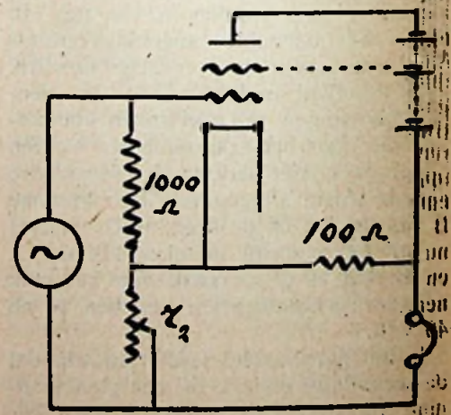
Figuur 7. — Bepaling van de steilheid S eener lamp. Wanneer r_2 wordt ingesteld op stilte in de telefoons, is (met een kleine verwaarloozing):
