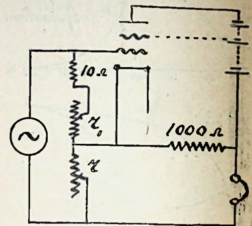
Figuur 6. — Bepaling van den inwendigen weerstand R_i . Wanneer r de zelfde waarde heeft, waarop die weerstand bij de meting volgens fig. 5 moest worden ingesteld en r_1 nu wordt ingesteld op stilte in de telefoons (of minimum geluid), is
