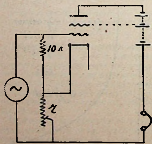
Figuur 5. — Meetinstallatie voor de bepaling van den versterkingsfactor g . Wanneer r zoo ingesteld wordt, dat de zoemertoon in de telefoon niet meer wordt gehoord, is
